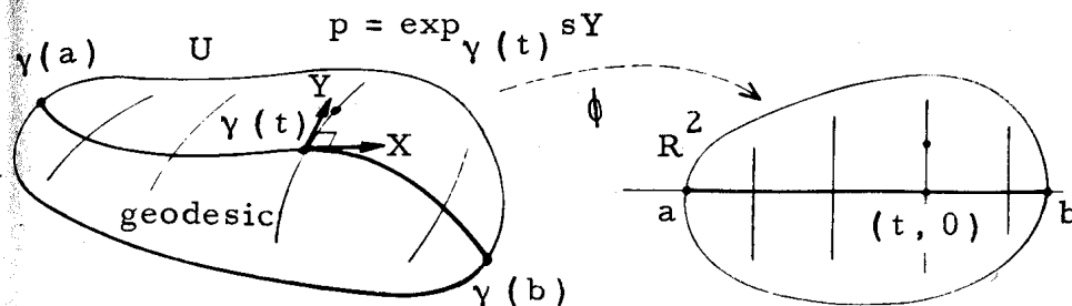
Fig. 9.1 Fermi Coordinates
